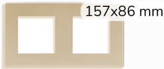
RP2_A 2-rámeček
