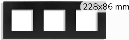
RP3_A 3-rámeček
